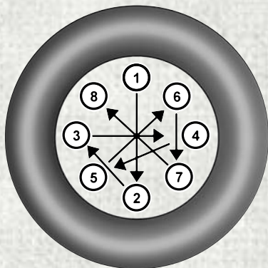
Séquence numérotée des écrous de roue (8)
