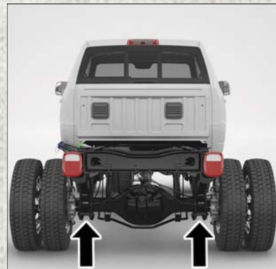
Emplacements de levage arrière
