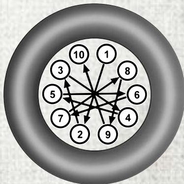
Séquence numérotée des écrous de roue (10)
